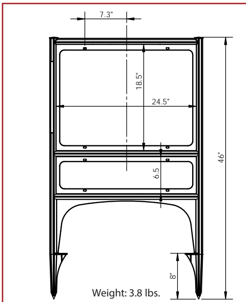
REALICADE DIMENSIONS
